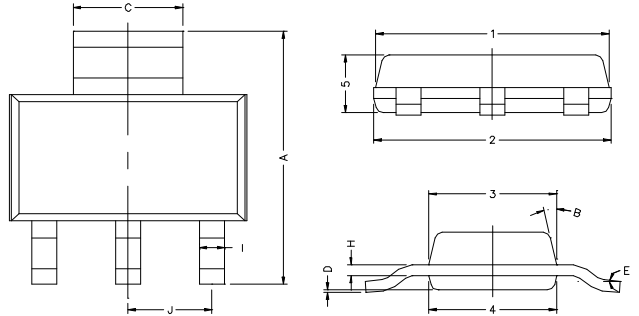
SOT-223
